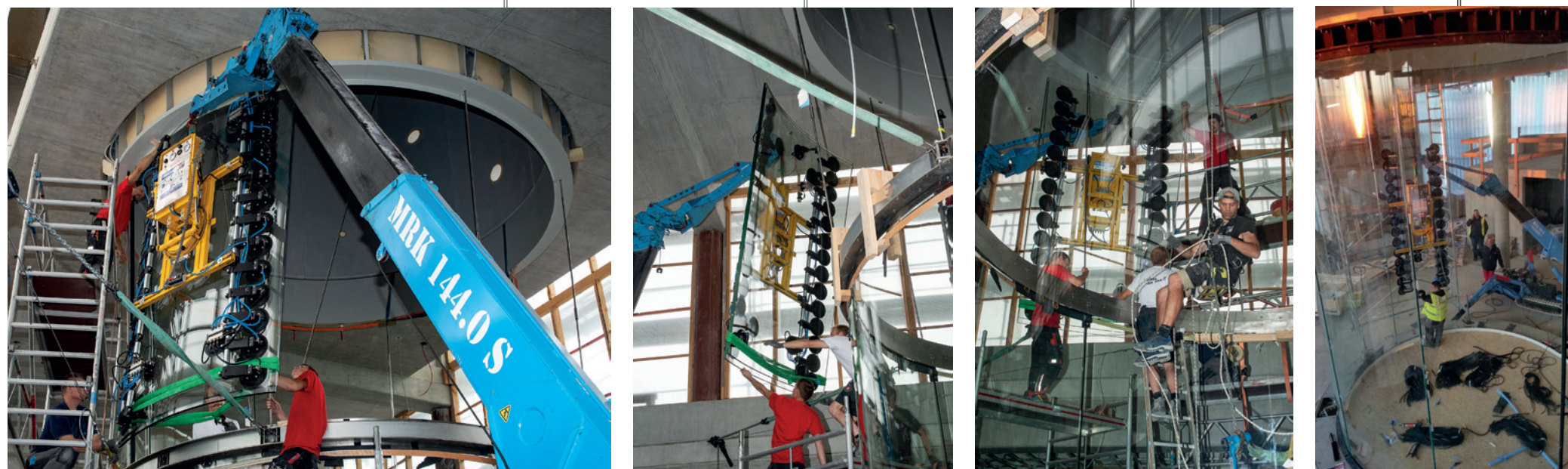
Macaraua de montaj MRK 144.0 S și instalația de aspirare cu vid VSG 1000 KR la vitrarea Flight Chamber
