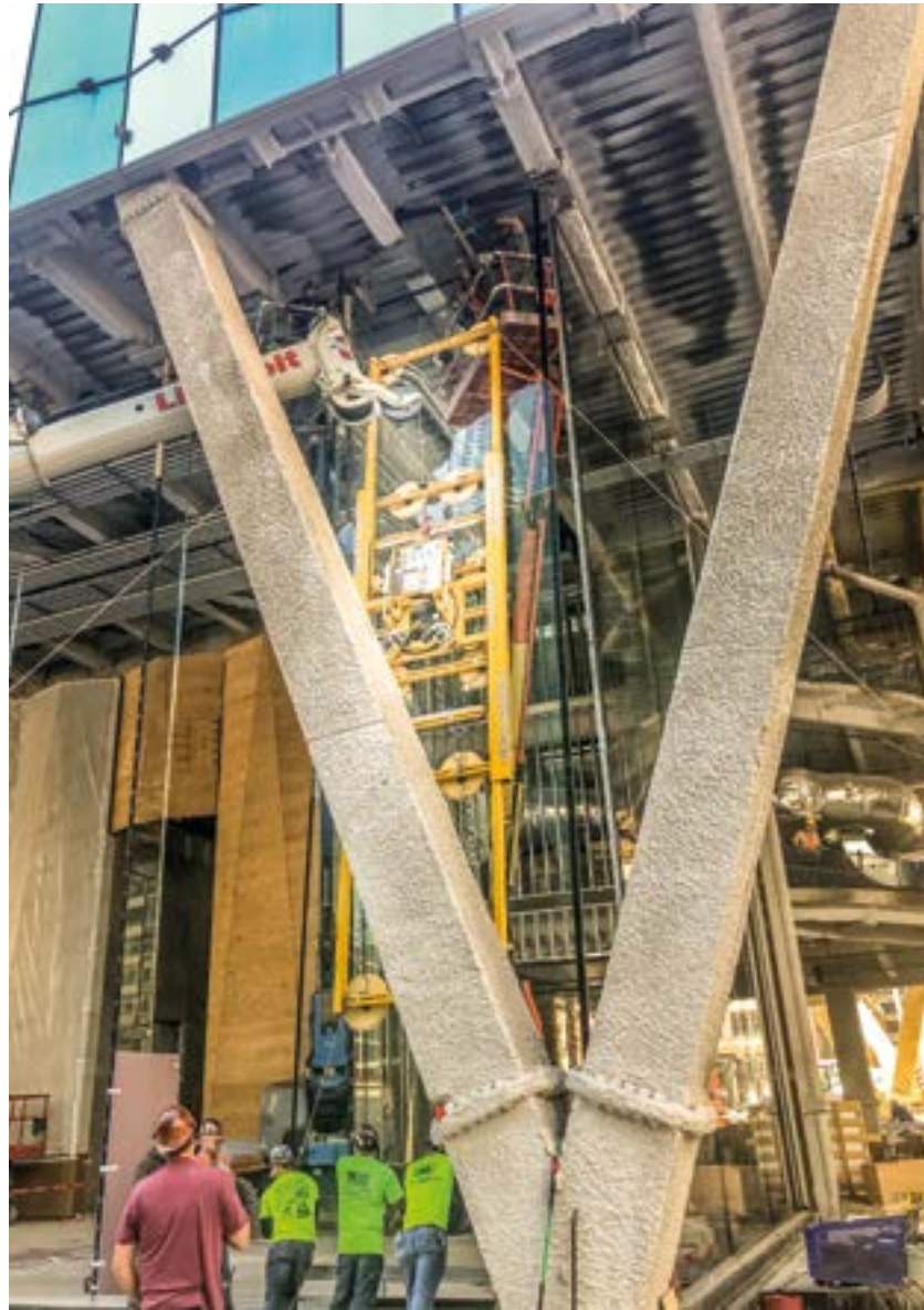
Das Scheibenelement wird mit modifizierter Glasmontage-Anlage hinter die Säule gehoben
