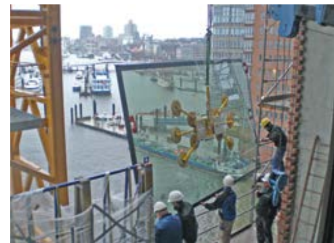
Montage der Panoramasscheiben mit dem MRK 86.0
